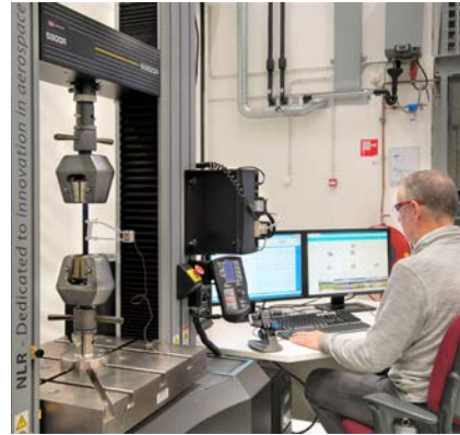
Instron 5882
